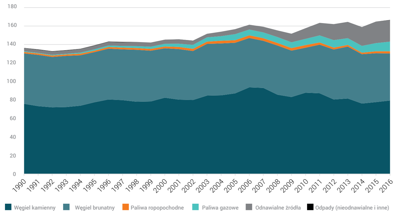
Rys. 25. Produkcja energii elektrycznej w Polsce w latach 1990-2016 [TWh]
