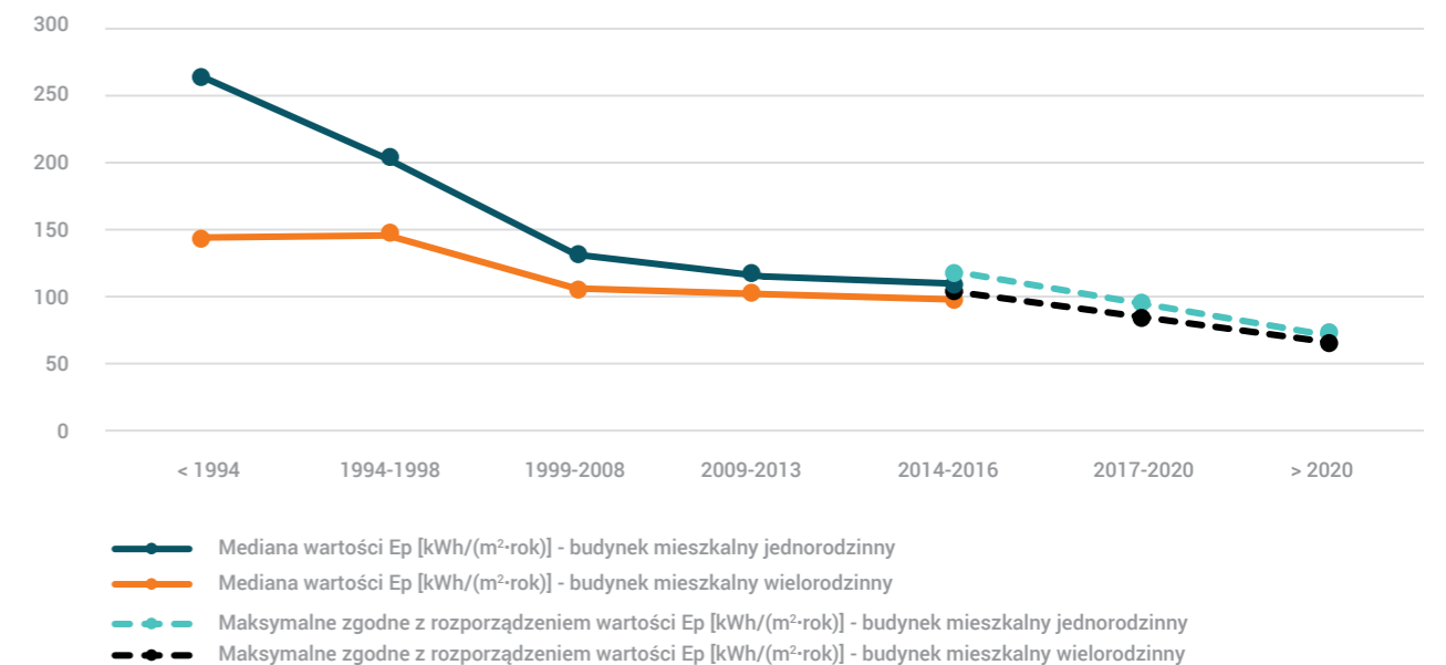
Rys. 24. Wartości wskaźnika rocznego zapotrzebowania na energię pierwotną budynków mieszkalnych w zależności od przeznaczenia oraz roku oddania do użytkowania Ep [kWh/(m²·rok)]
